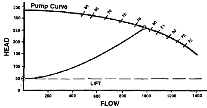
(d) Interpolate system curve
